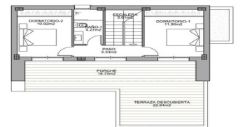
PLANTA PRIMERA
